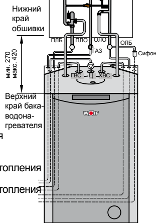
Трубы при открытой установке
